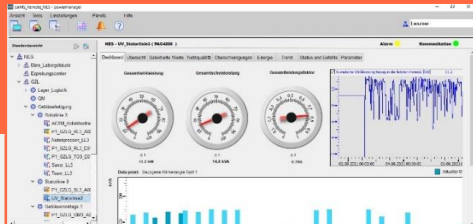
Selbstlernende Algorithmen
